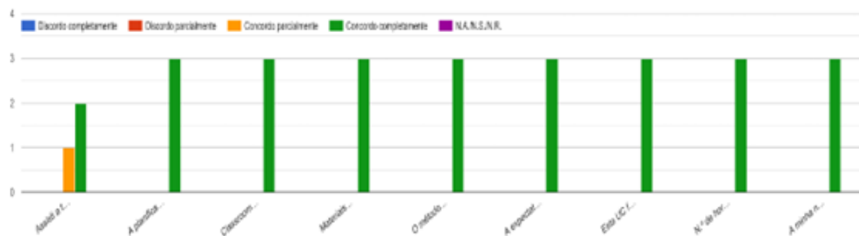
Matemática II (Mat II)
