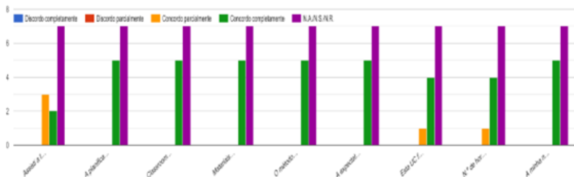
Estatística Descritiva (ED)
