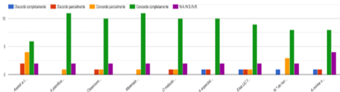
Estatística Descritiva (ED)
